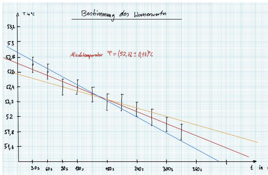
Abbildung 3.1: Diagramm zur Bestimmung des Wasserwertes des Kalorimeters
